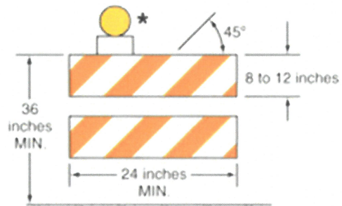
TYPE 2 BARRICADE **
