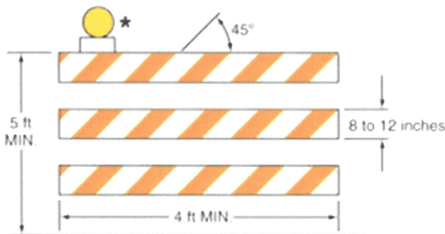
TYPE 3 BARRICADE **
