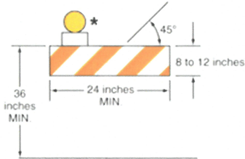
TYPE 1 BARRICADE **
